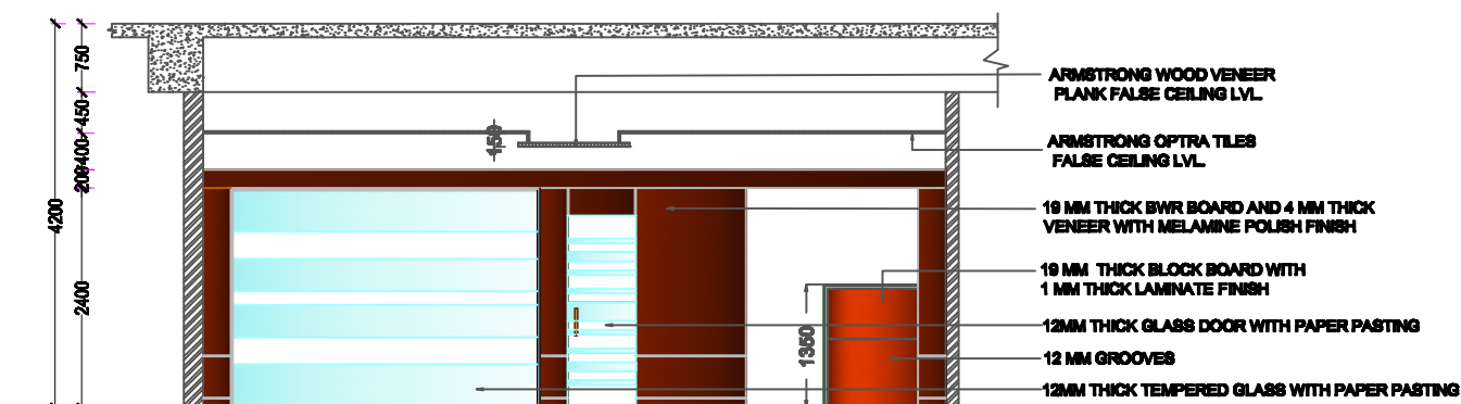
ELEVATION G
